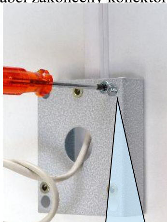
1. instalace montážního držáku – čtyřmi šrouby na zeď
