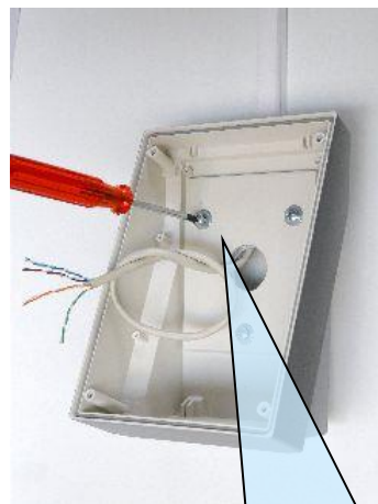
3. Montáž zadní části krabice terminálu k držáku - třemi šrouby (jsou součástí držáku).
